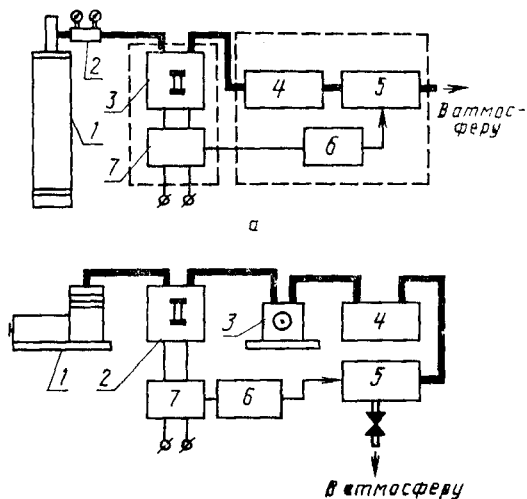
Блок-схемы приборов для измерения массовой доли газов:
